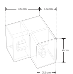
ILUCONWS90HT IP 20 Cople de 90°, mecánico y electrificado, policarbonato transparente, para luminarios de la serie ILUINTWS, conexión horizontal.
