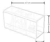
ILUCONWS180HT IP 20 Cople lineal de 180°, mecánico y electrificado, policarbonato transparente, para luminarios de la serie ILUINTWS, conexión horizontal.
