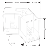
ILUCONWS120HT IP 20 Cople de 120°, mecánico y electrificado, policarbonato transparente, para luminarios de la serie ILUINTWS, conexión horizontal.
