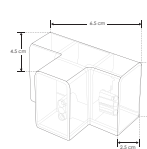
ILUCONWS120HT IP 20 Cople en forma de T, mecánico y electrificado, policarbonato transparente, para luminarios de la serie ILUINTWS, conexión horizontal.
